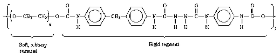
Fig: Chemical
